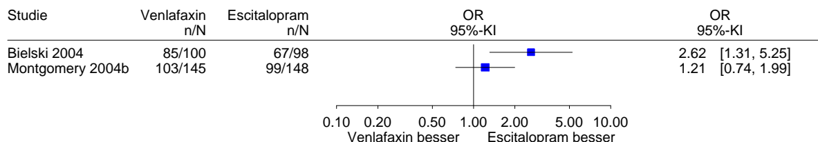
Abbildung 123: Meta-Analyse UEs, Venlafaxin vs. Escitalopram, Kurzzeit-Akutstudien
