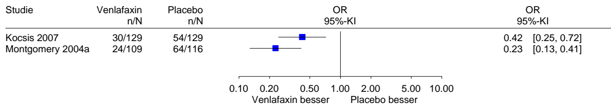
Abbildung 106: Meta-Analyse Rezidivrate, Venlafaxin vs. Placebo, Langzeitstudien, Definition 1
