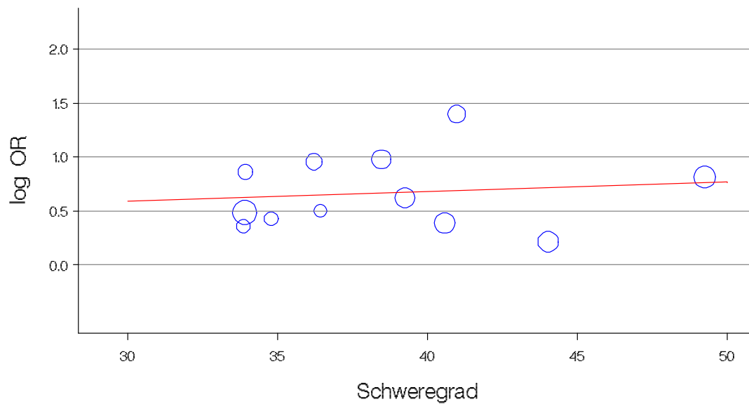
Abbildung 196: Meta-Regression Schweregrad, Duloxetin vs. Placebo, Ansprechens (Steigungsparameter: 0,0089; p = 0,67 (Interaktionstest))
