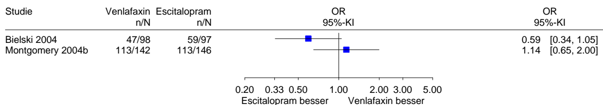
Abbildung 79: Meta-Analyse Ansprechen, Venlafaxin vs. Escitalopram, Kurzzeit-Akutstudien
