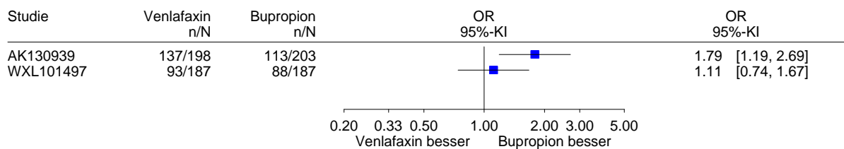
Abbildung 127: Meta-Analyse UEs, Venlafaxin vs. Bupropion, Kurzzeit-Akutstudien
