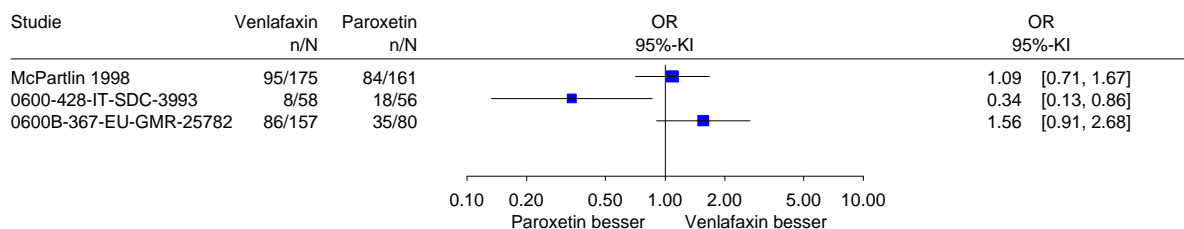
Abbildung 67: Meta-Analyse Remission, Venlafaxin vs. Paroxetin, Kurzzeit-Akutstudien
