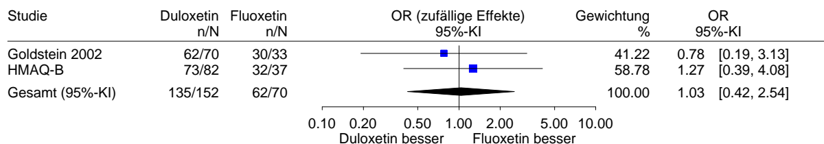
Abbildung 43: Meta-Analyse UEs, Duloxetin vs. Fluoxetin, Kurzzeit-Akutstudien
