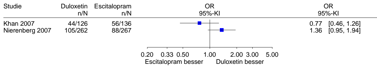
Abbildung 6: Meta-Analyse Remission, Duloxetine vs. Escitalopram, Kurzzeit-Akutstudien
