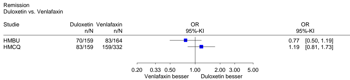
Abbildung 163: Meta-Analyse Remission, Duloxetin vs. Venlafaxin, Direktvergleich
