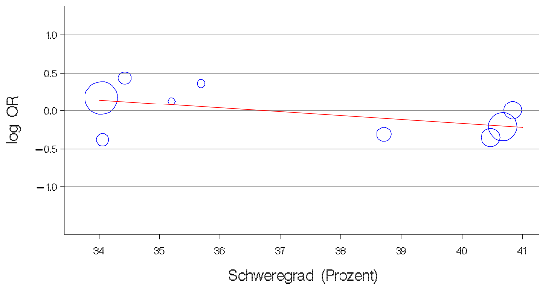
Abbildung 199: Meta-Regression Schweregrad, Duloxetin vs. SSRI, Ansprechen (Steigungsparameter: -0,0426; p = 0,13 (Interaktionstest))
